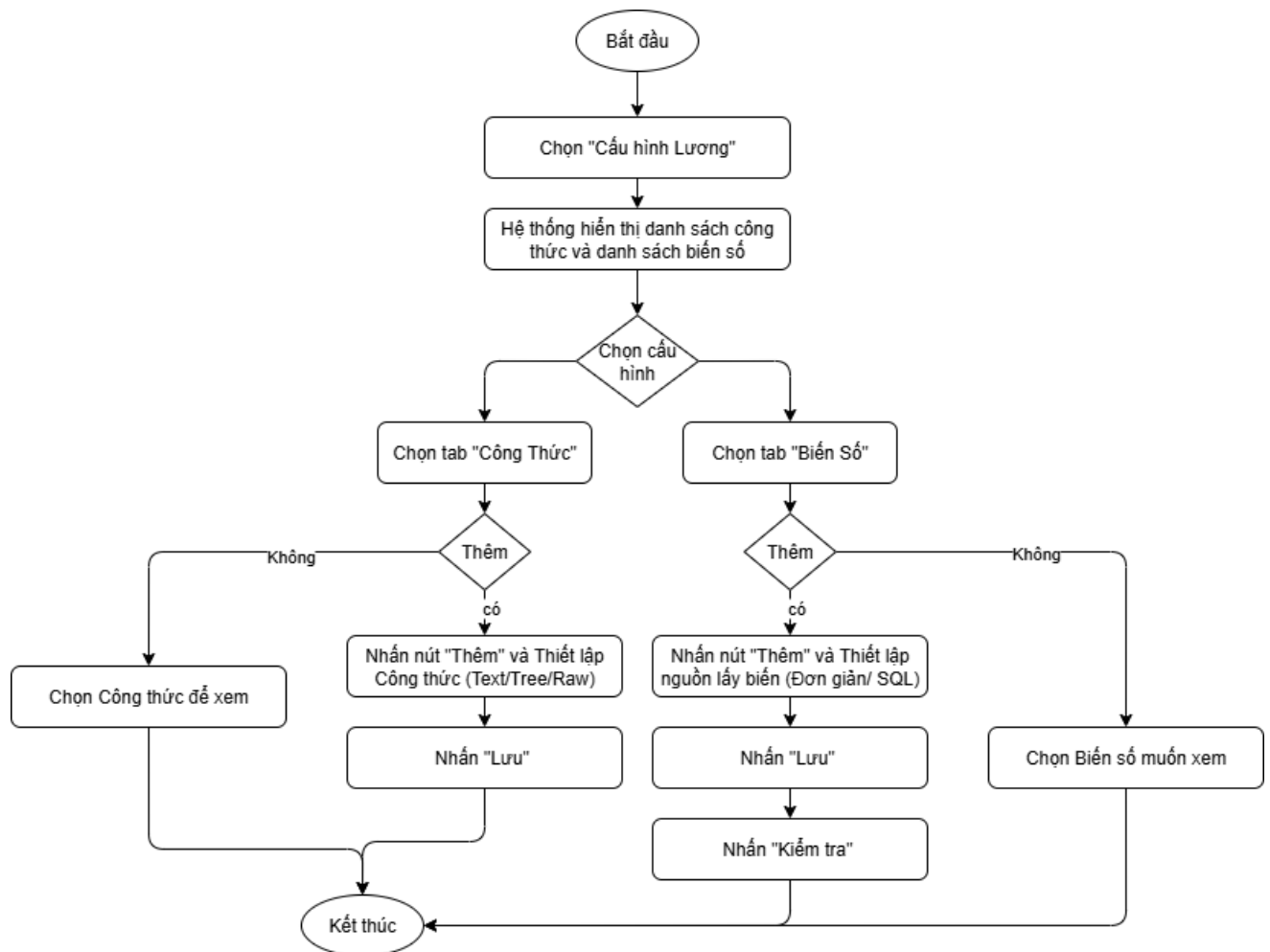
Hình 2-21: Sơ đồ quy trình Cấu hình lương.
