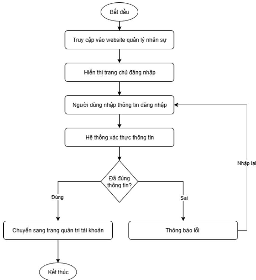
Hình 2-8: Sơ đồ quy trình Đăng nhập.
