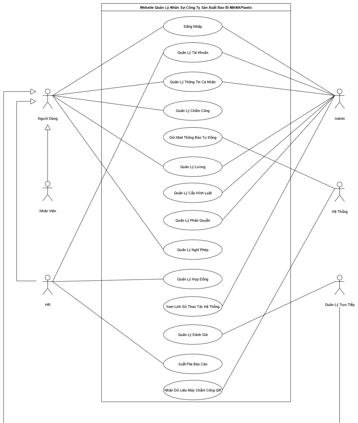
Hình 2-33: Sơ đồ use case tổng quát
