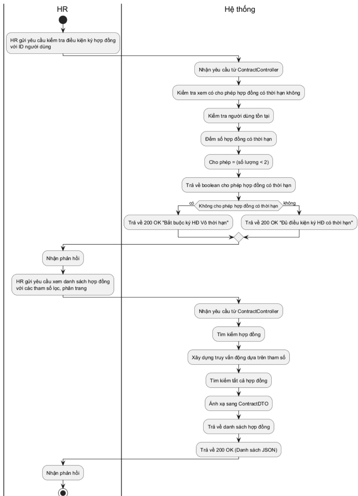
Hình 3-61: Sơ đồ hoạt động xem & kiểm tra hợp đồng.
