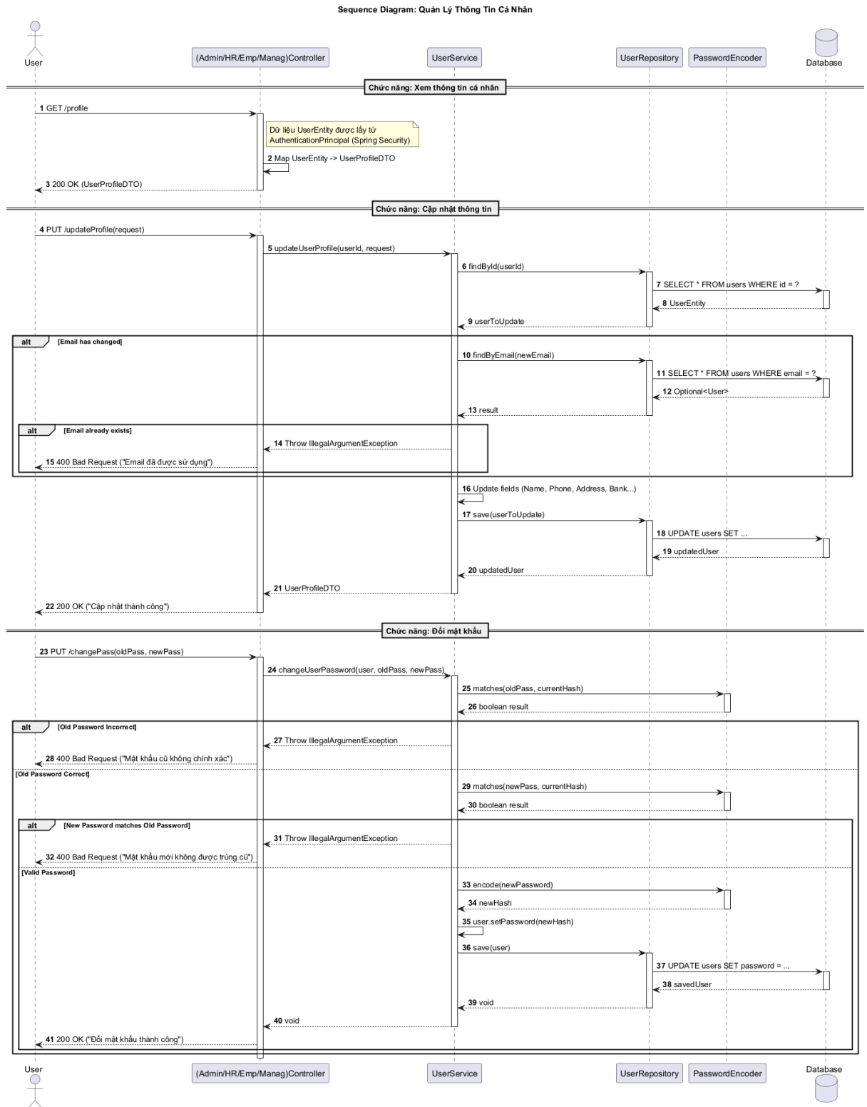
Hình 3-24: Sơ đồ tuần tự quản lý thông tin cá nhân.
