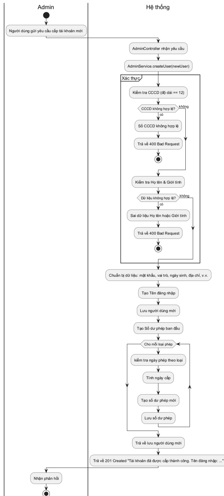
Hình 3-49: Sơ đồ hoạt động cấp tài khoản.
