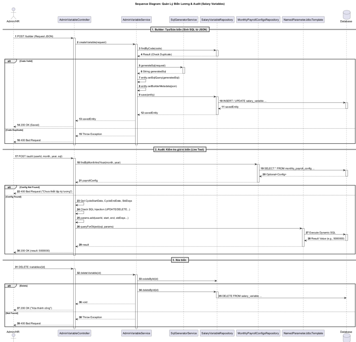
Hình 3-39: Sơ đồ tuần tự cấu hình biến đầu vào tính lương.
