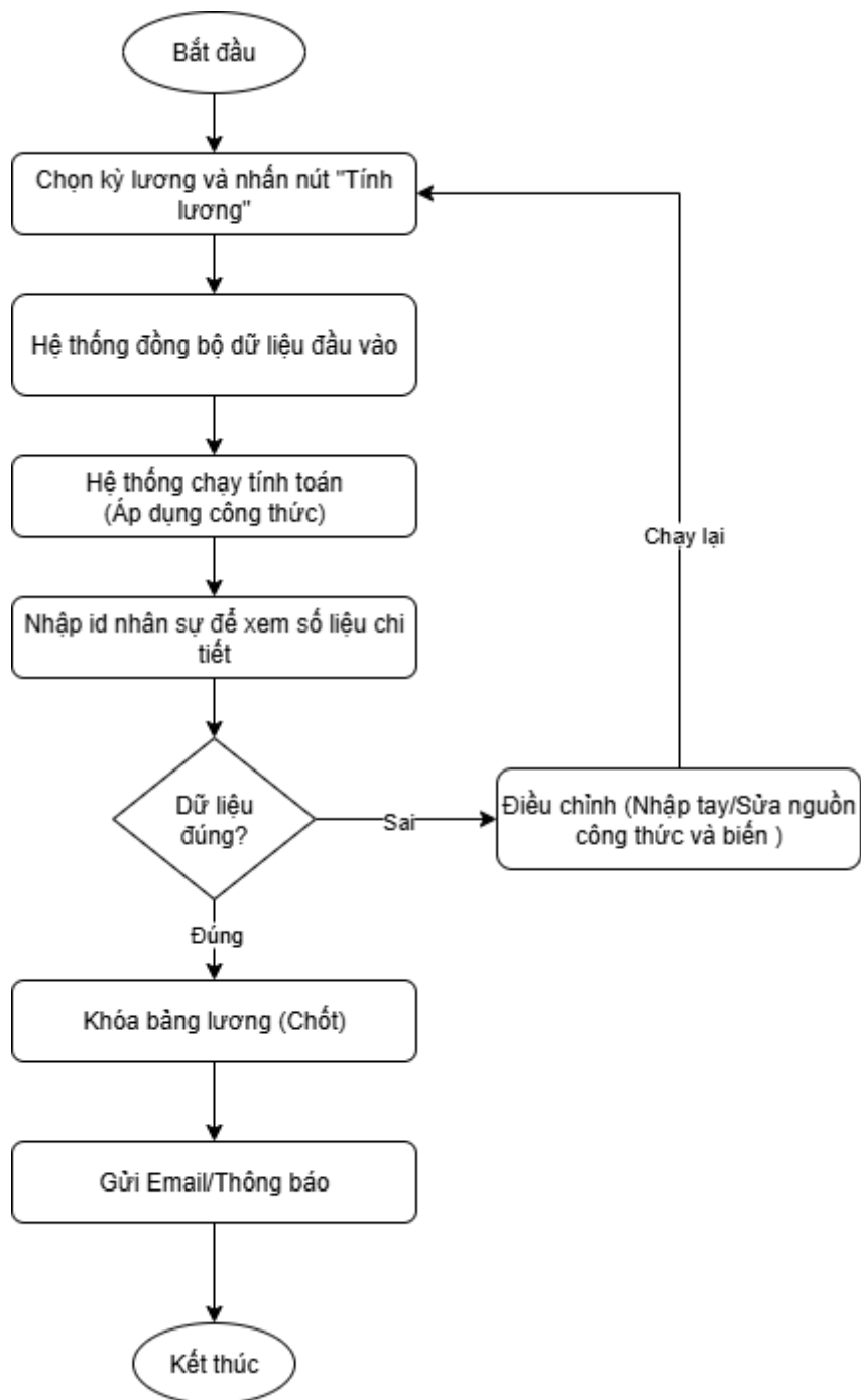
Hình 2-22: Sơ đồ quy trình Tính lương.
