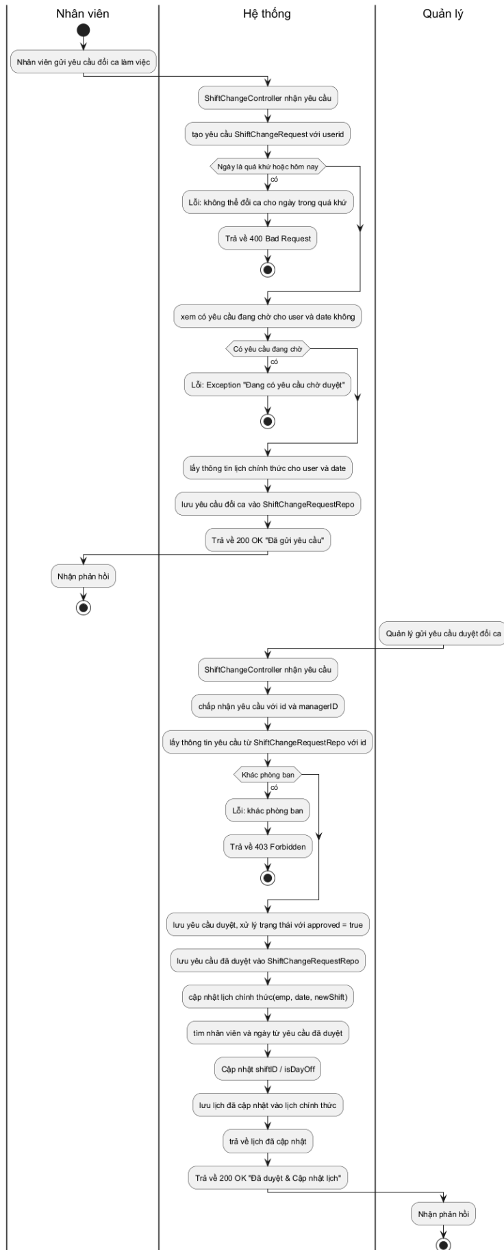
Hình 3-57: Sơ đồ hoạt động đăng ký đổi ca lịch làm việc.
