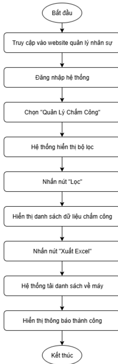
Hình 2-17: Sơ đồ quy trình Xuất file báo cáo dữ liệu chấm công.
