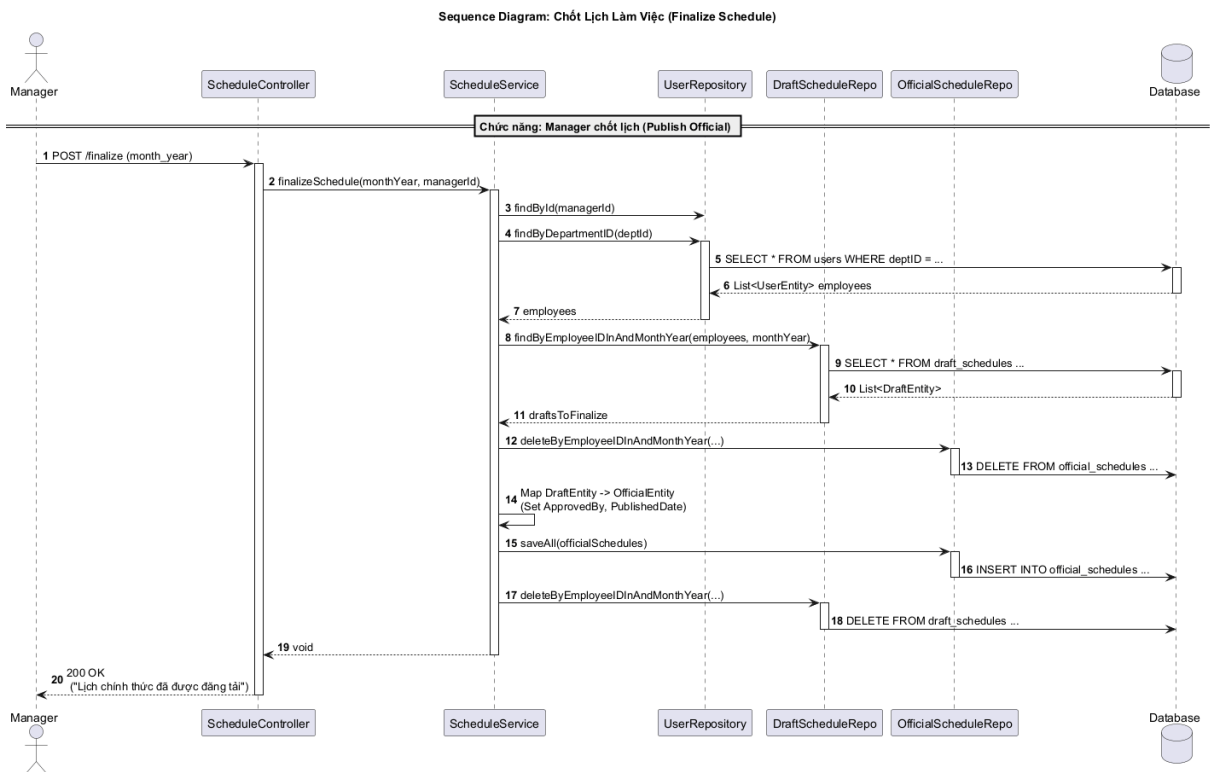
Hình 3-30: Sơ đồ tuần tự lịch chính thức (Office).
