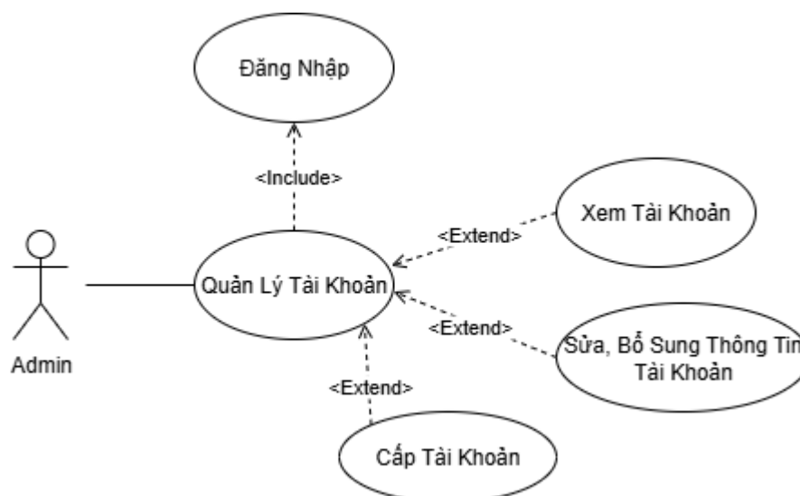
Hình 3-9: Use case quản lý tài khoản - Admin.
