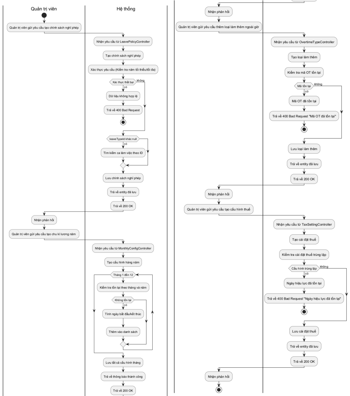
Hình 3-48: Sơ đồ hoạt động cấu hình luật lao động.
