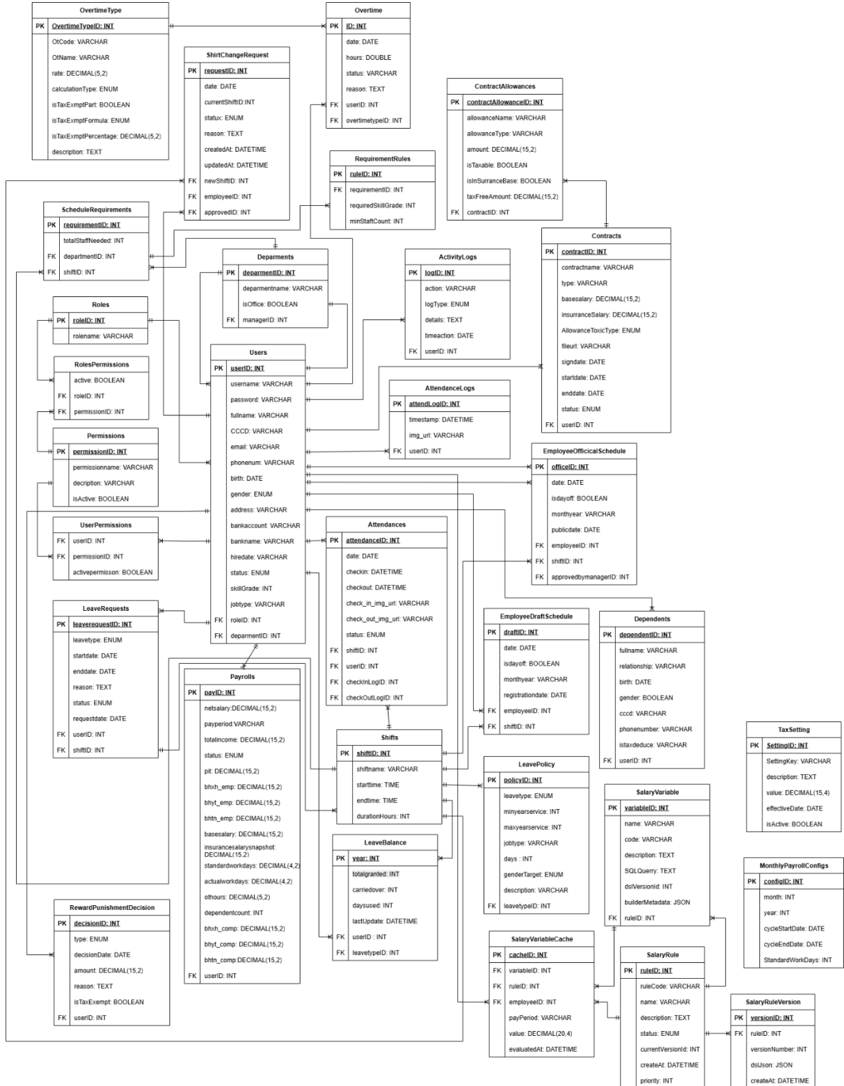
Hình 3-1: Mô hình dữ liệu vật lý
