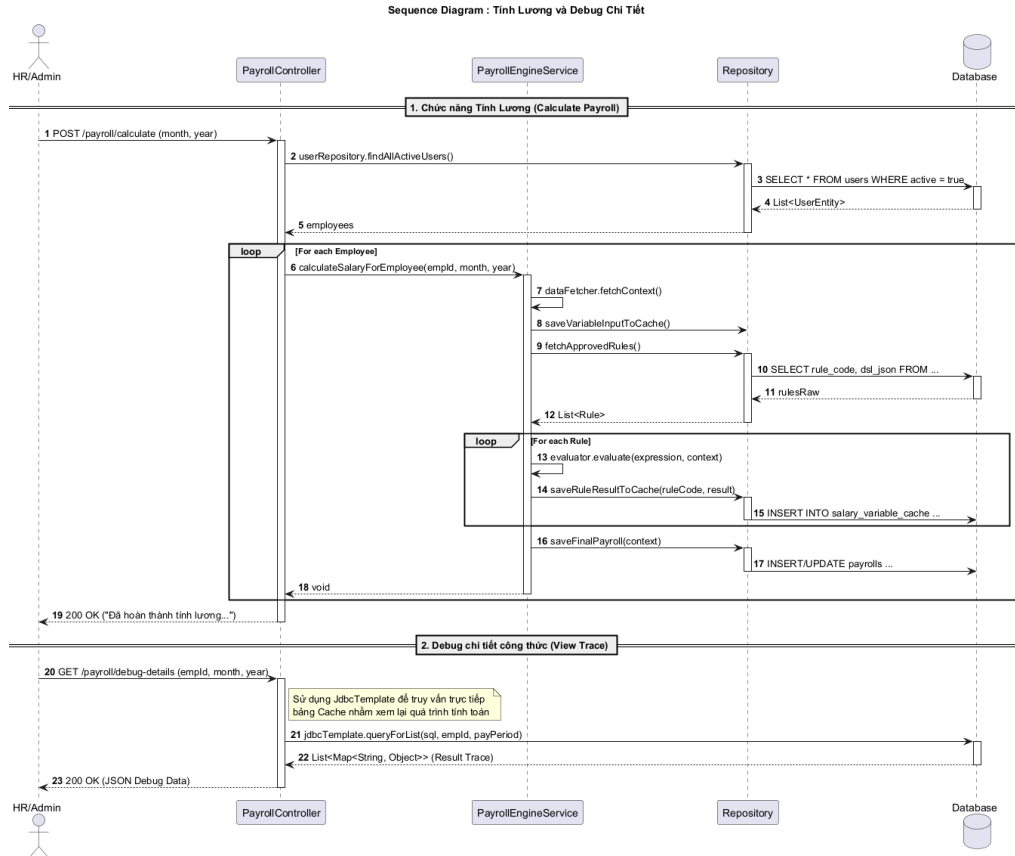
Hình 3-37: Sơ đồ tuần tự xem quá trình & tính lương.
