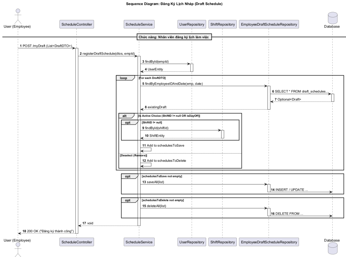
Hình 3-29: Sơ đồ tuần tự lịch nháp (Draft).
