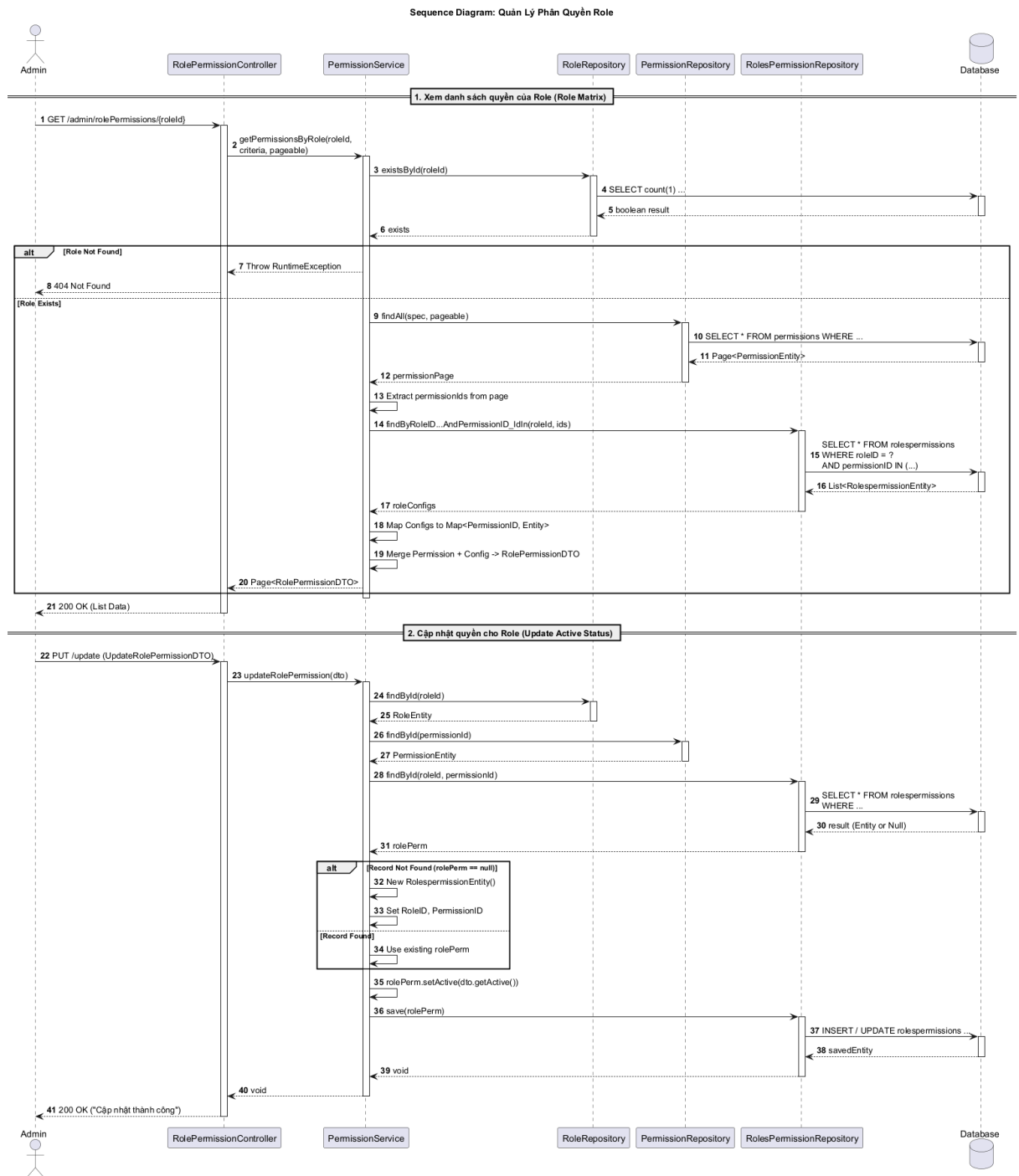
Hình 3-25: Sơ đồ tuần tự phân quyền chức năng vai trò (Role).
