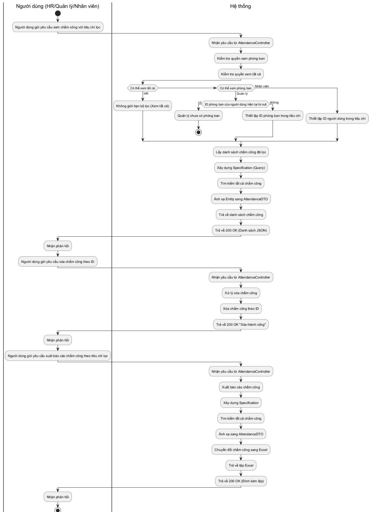
Hình 3-54: Sơ đồ hoạt động quản lý chấm công.
