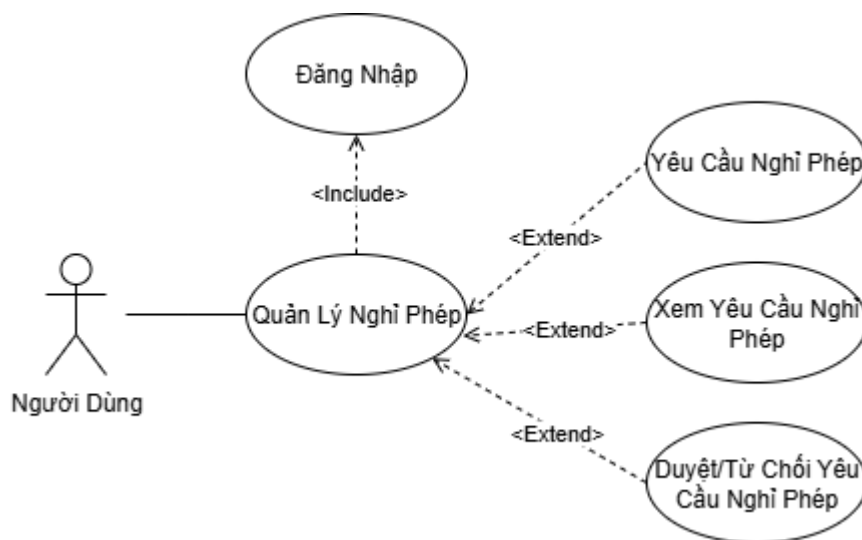
Hình 3-4: Use case quản lý nghỉ phép.
