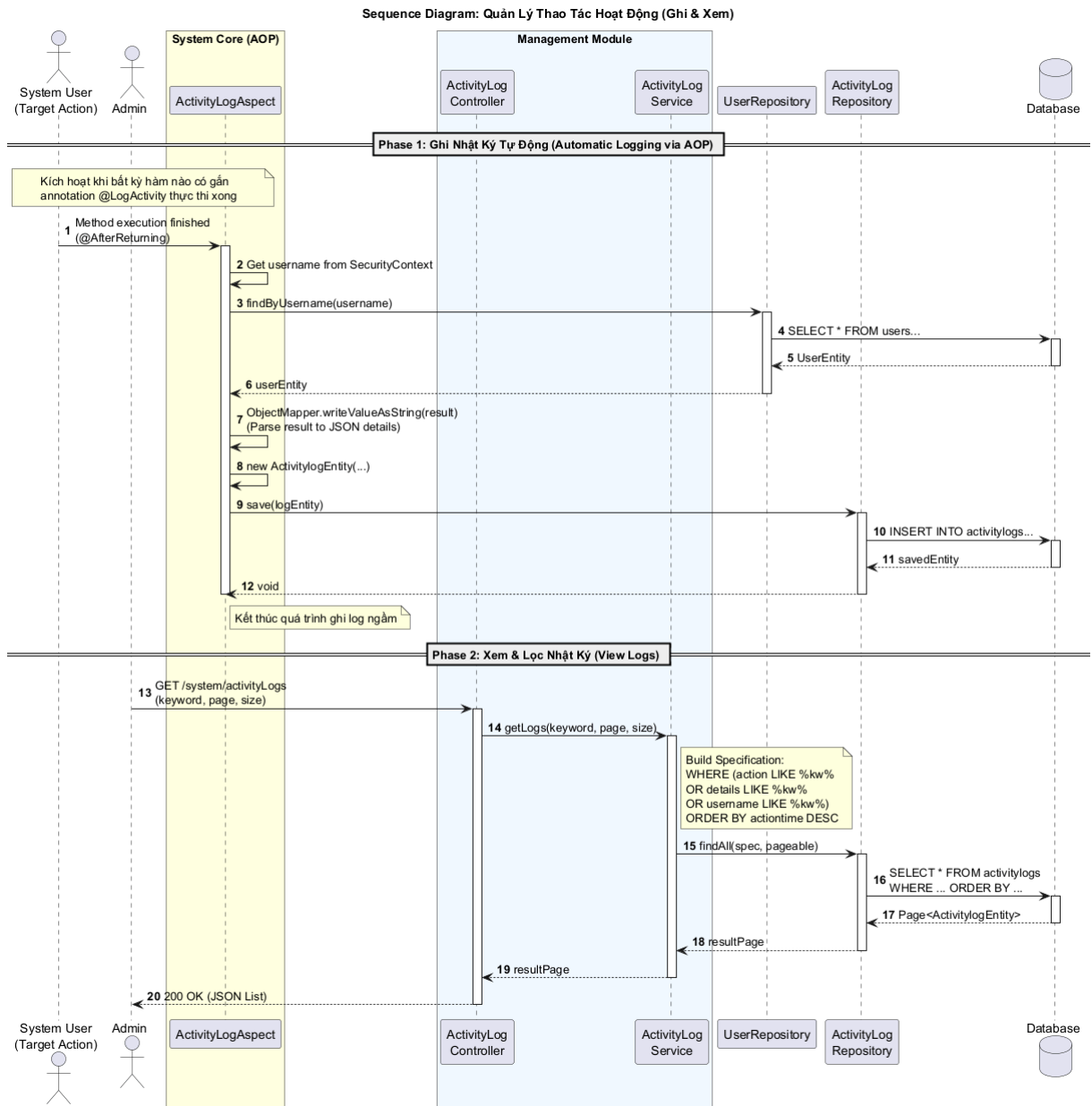
Hình 3-41: Sơ đồ tuần tự ghi log & xem log các hoạt động trong hệ thống.
