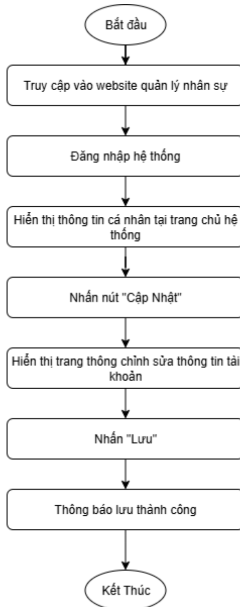
Hình 2-10: Sơ đồ quy trình Quản Lý Thông Tin Cá Nhân.
