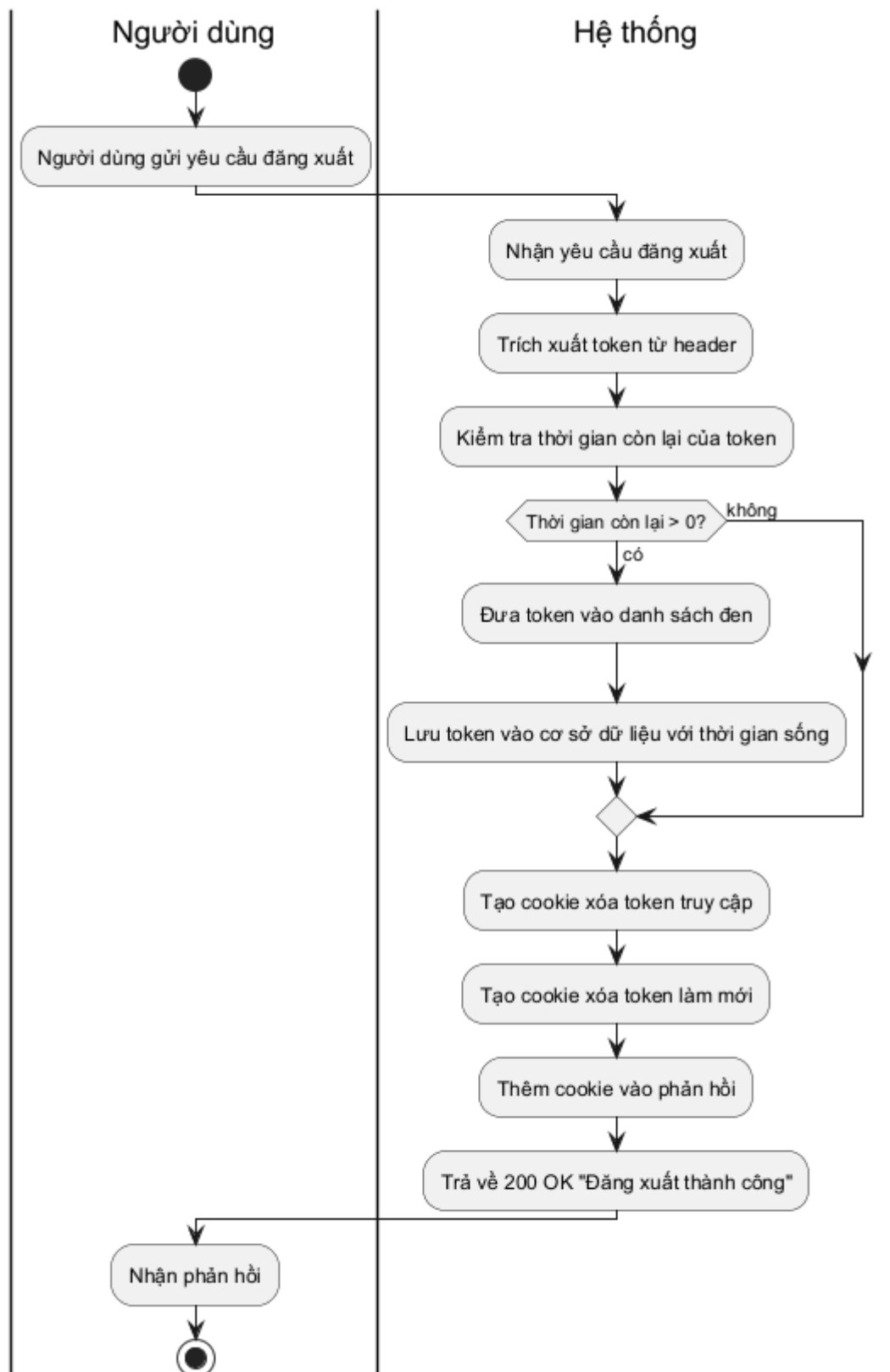
Hình 3-43: Sơ đồ hoạt động đăng xuất.
