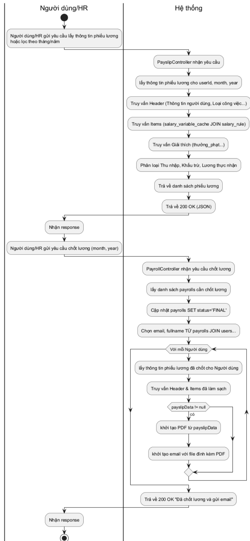
Hình 3-50: Sơ đồ hoạt động xem & mail phiếu lương.
