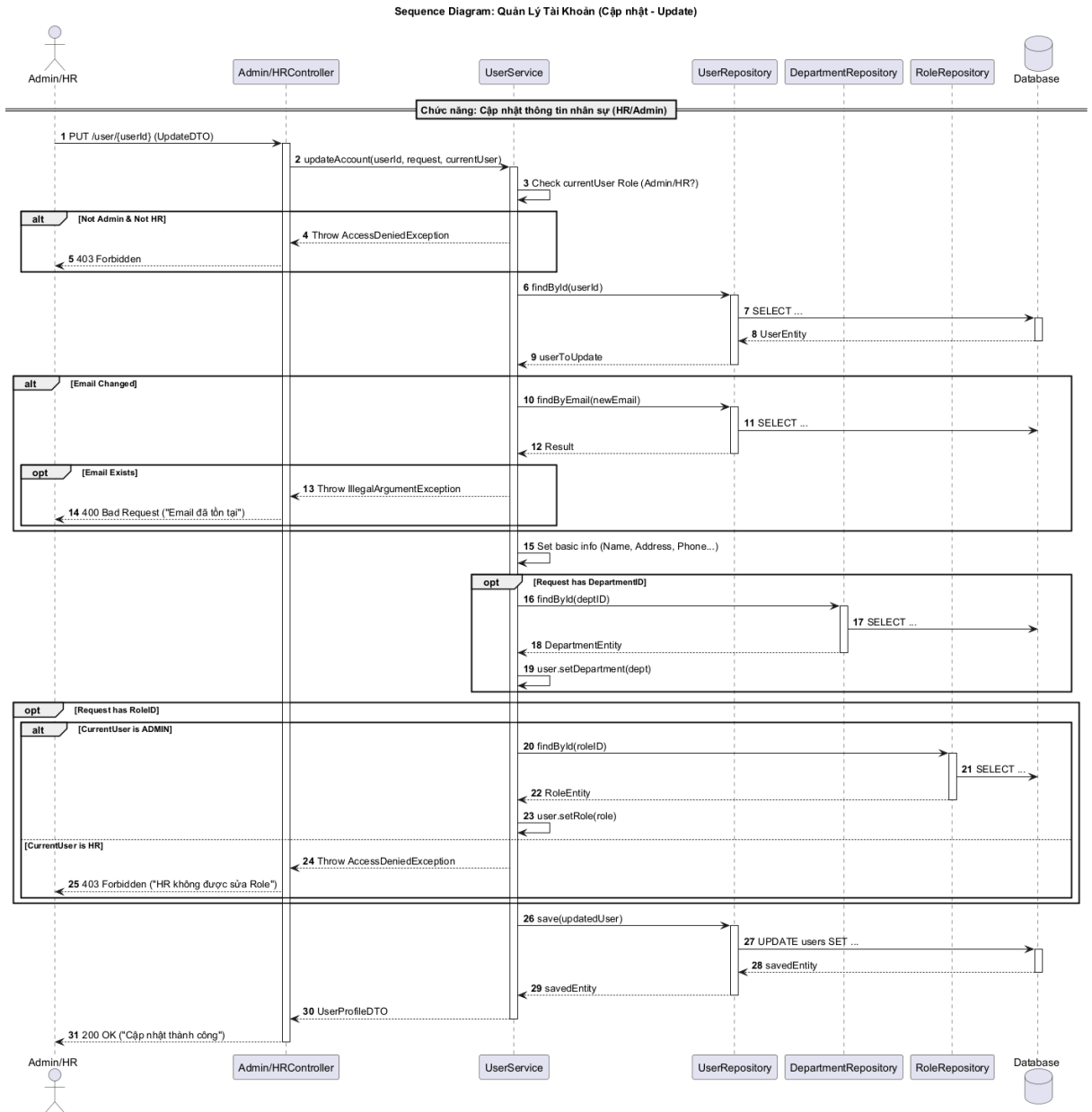
Hình 3-23: Sơ đồ tuần tự cập nhật tài khoản.
