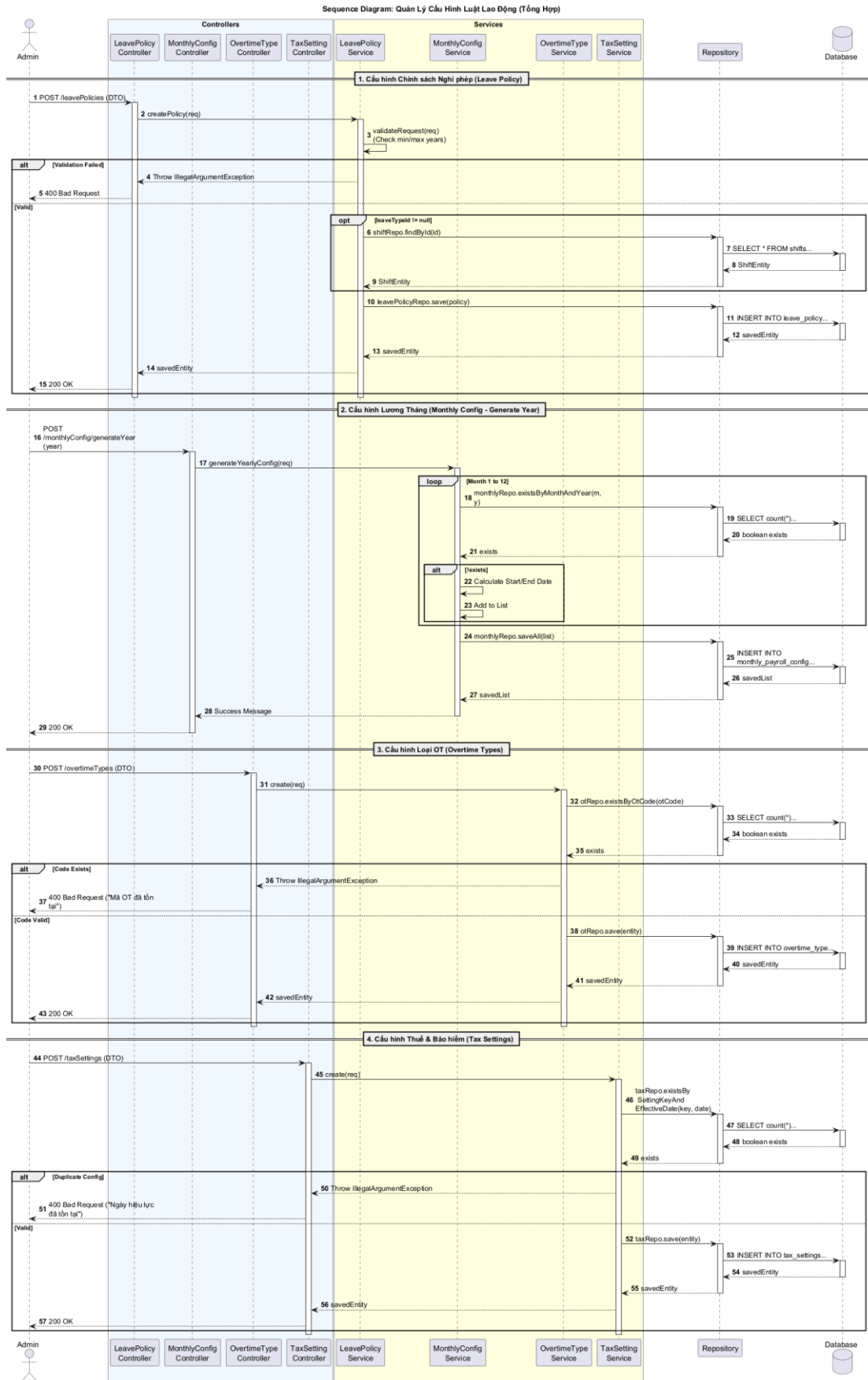
Hình 3-32: Sơ đồ tuần tự quản lý cấu hình luật lao động.
